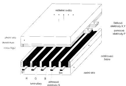
Řez výškem plasmového zobrazovače
