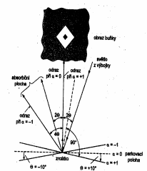
Odraz světla ze zdroje pro různá vychýlení zrcátka buňky matice DMD
