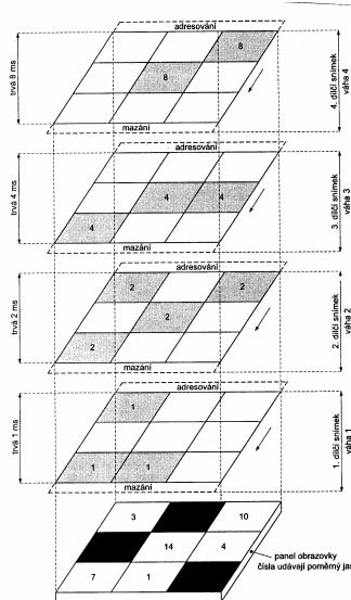
Příklad vytváření 16 úrovní jasu v devíti buňkovém obrazovém bodu matice DMD pomocí časové sekvence čtyř kryjících se obrazových polí s dobou trvání klesající dle geometrické řady.
