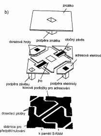
Struktura jedné buňky DMD
